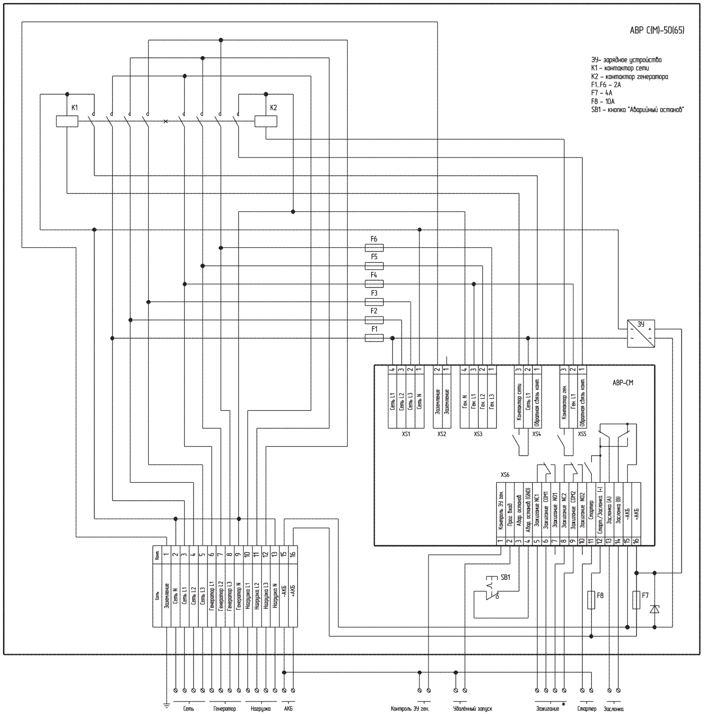
Рис 6.3. Пример схемы подключения контроллера ABP С(М)-50(65) для конфигурации AVR33
